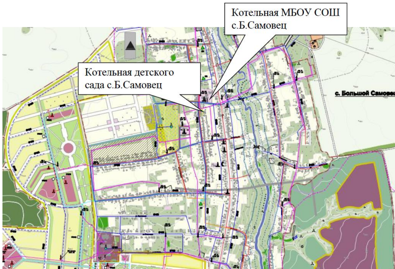
Рисунок 1. Зоны действия котельных
